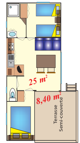
Modèle IRM Loggia 4 à 6 personnes - 25 m² + 8,40 m²
