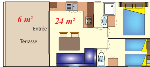
Modèle Louisiane Méditerranée Max. 4 personnes • 24 m² + 6 m² - 2 chambres
